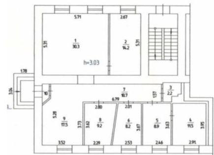
ПЛАН ПОМЕЩЕНИЙ
