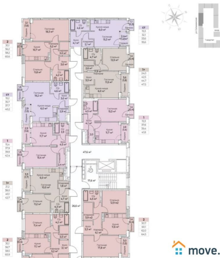
СЕКЦИЯ № 6 5 ЭТАЖ
